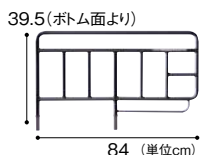
ベッドサイドレール K-173
