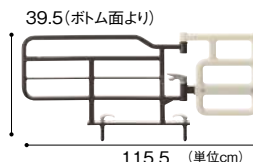
回転式アーム介助バー K-55R
