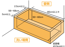
バスリフトの設置可否を判断する浴室の寸法
